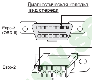
Колодка МК вид спереди, со стороны контактов
