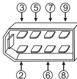
Колодка МК вид спереди, со стороны контактов
